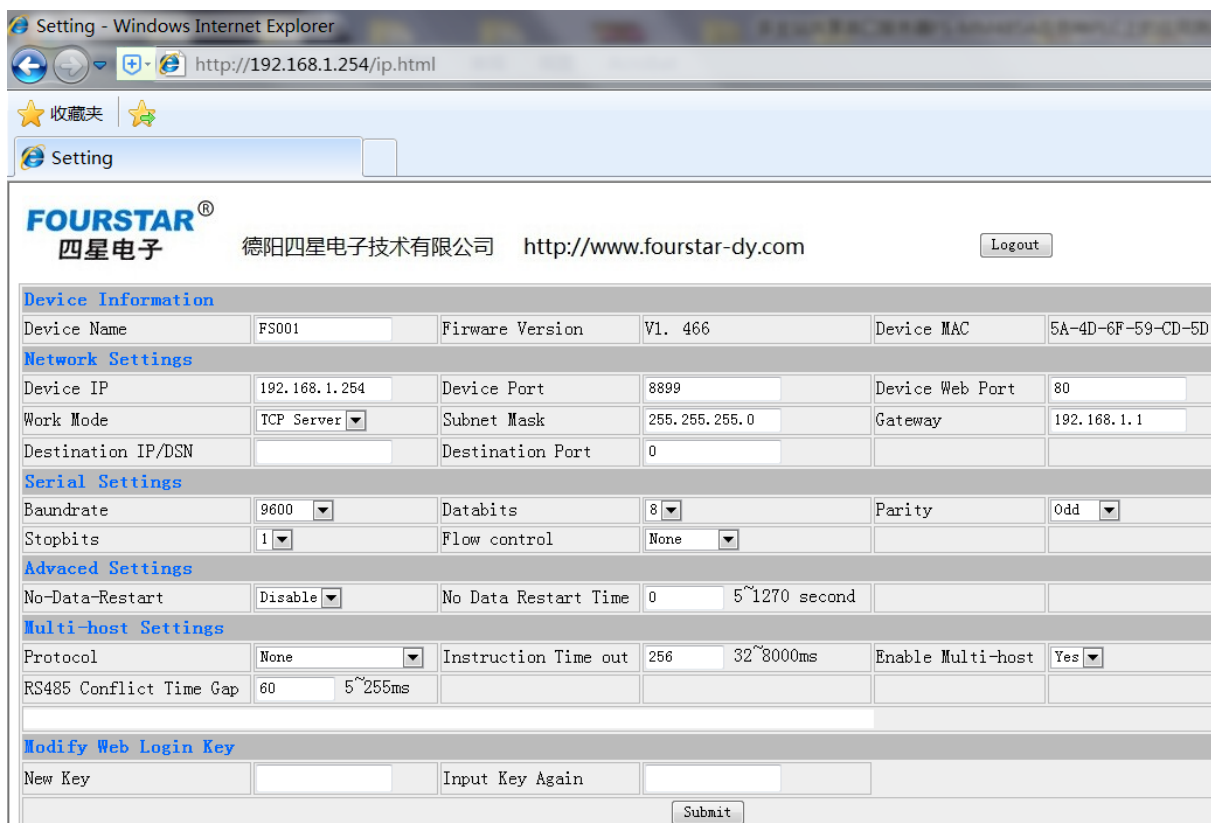
图 2 FS-ETH-Q 参数设置截图
