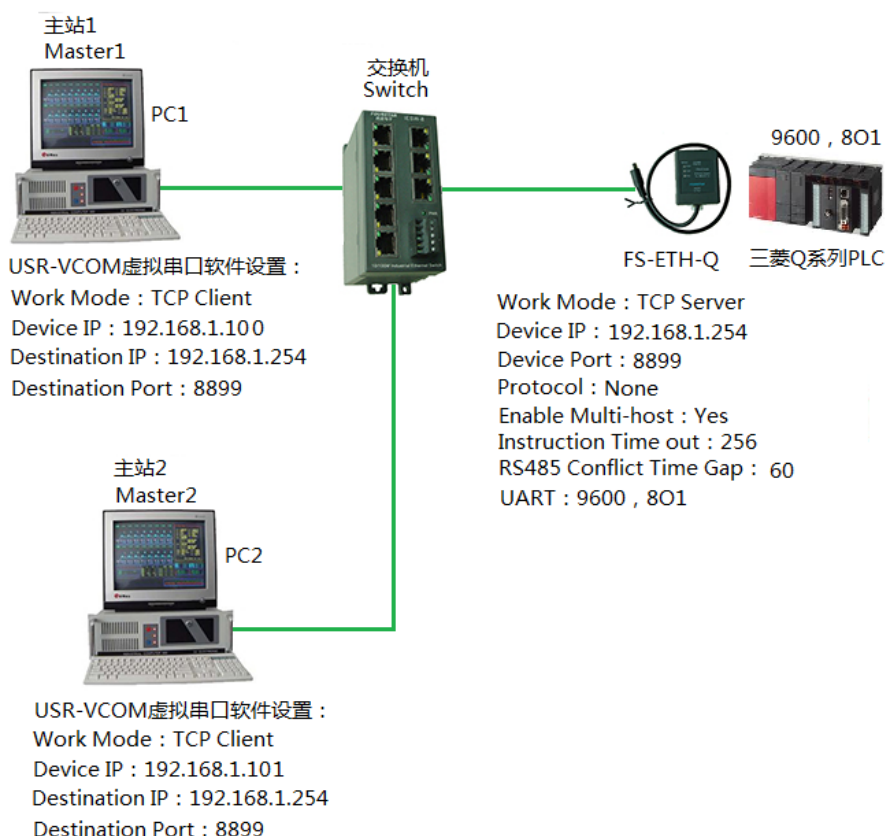
图 1 组态王与三菱 Q 系列 PLC 多主站通讯连接拓扑
