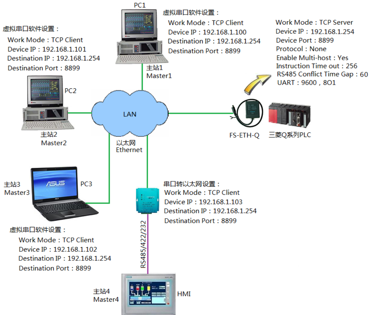
图5.2-2 多主站无协议透传通讯网络连接拓扑
