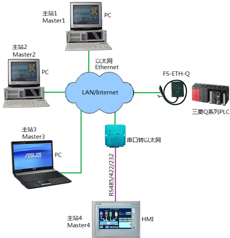
图 1-2 采用 FS-ETH-Q 的多主站通讯网络拓扑
