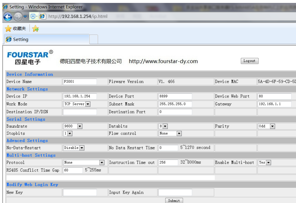
图5.2-1 FS-ETH-Q作多主站共享串口服务器时的设置
