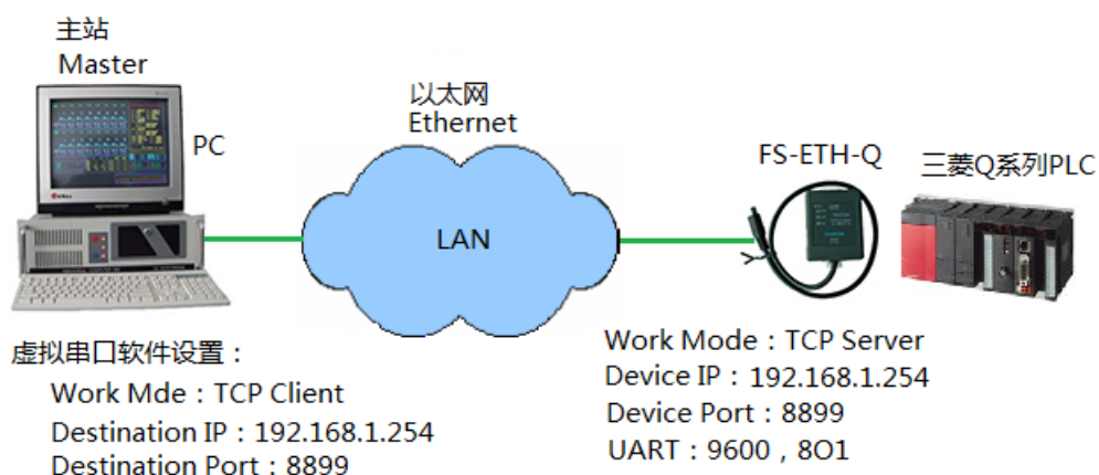
图5.1-1 计算机与Q系列PLC通过以太网通讯
