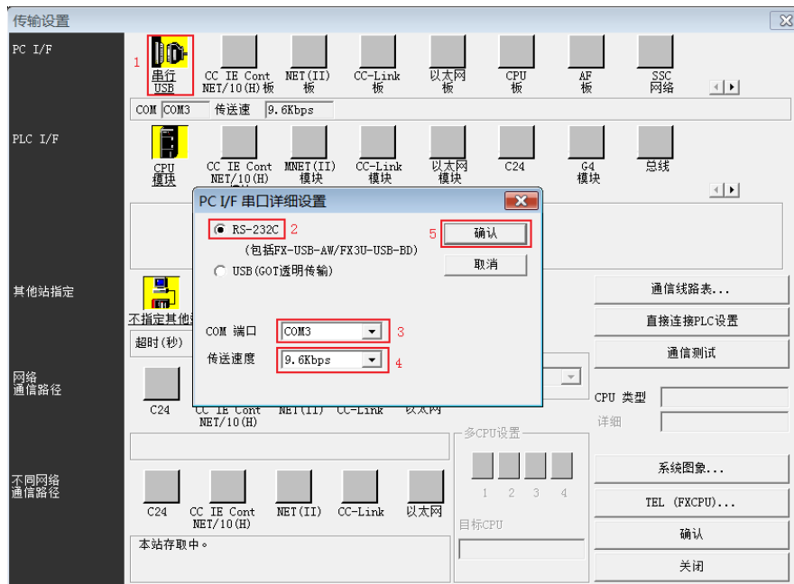
图 5.1-3 三菱 GX Developer 编程软件 的设置
