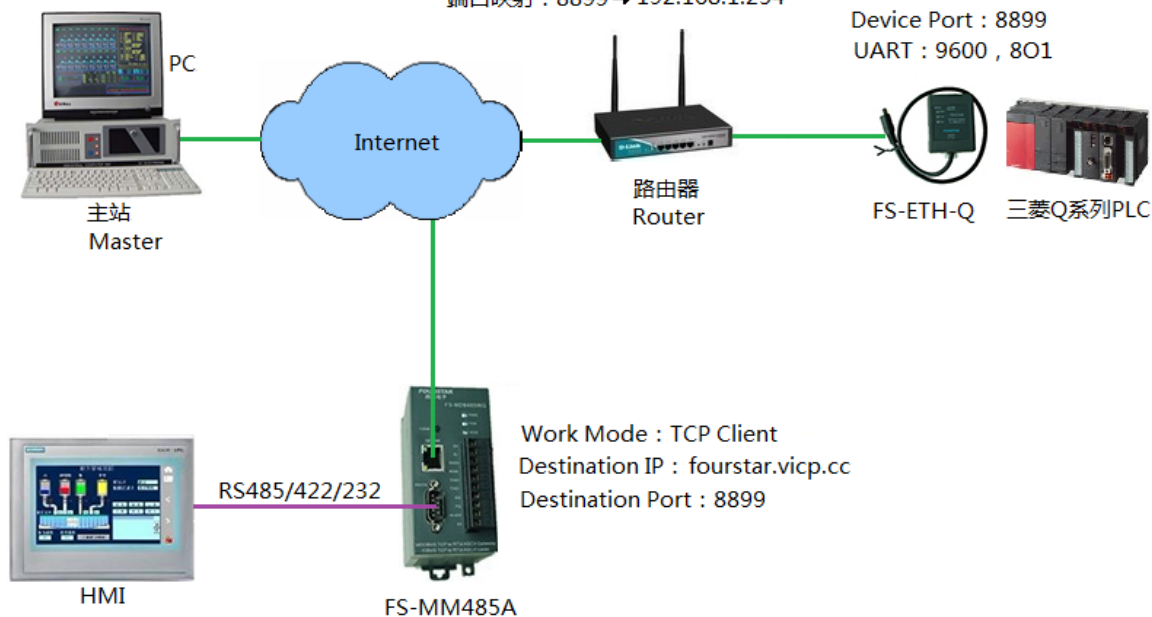
图5.3-1 FS-ETH-Q在互联网上的通讯网络拓扑
