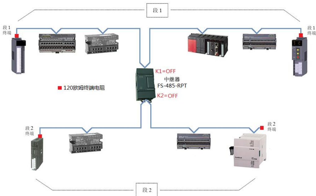
图 6-3 用 FS-485-RPT 中继器桥接总线
