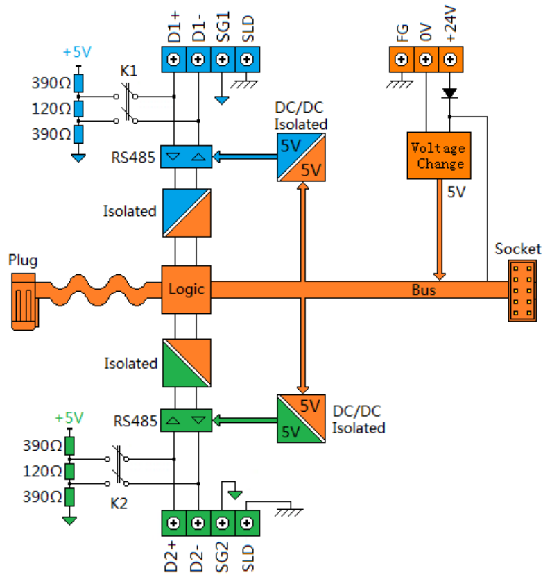
图 5-1 四星电子 FS-485-RPT 中继器集线器原理框图
