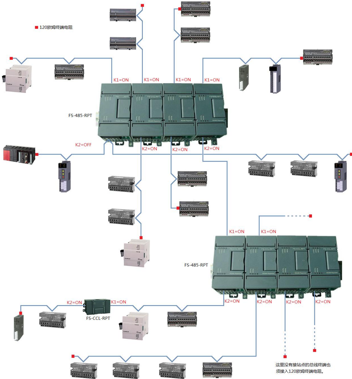
图 6-5 FS-485-RPT 级连
