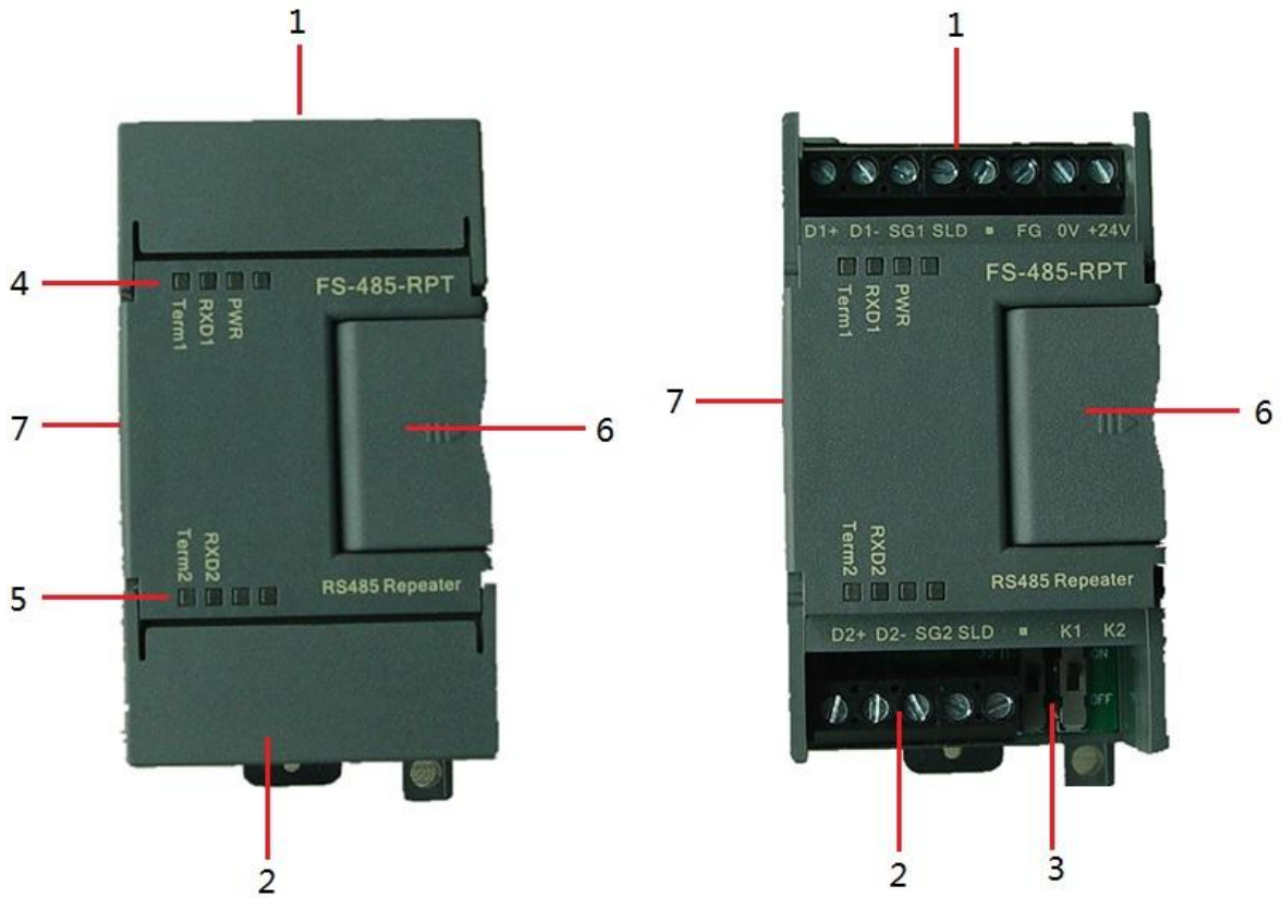
图 4-1 四星电子 FS-485-RPT 中继器集线器外形图
