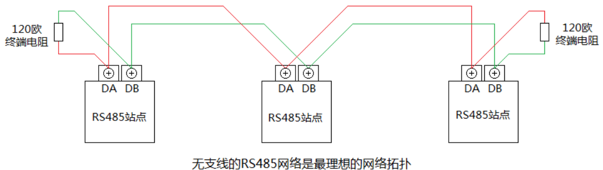
图1-2 RS485网络的干线、支线、终端电阻
