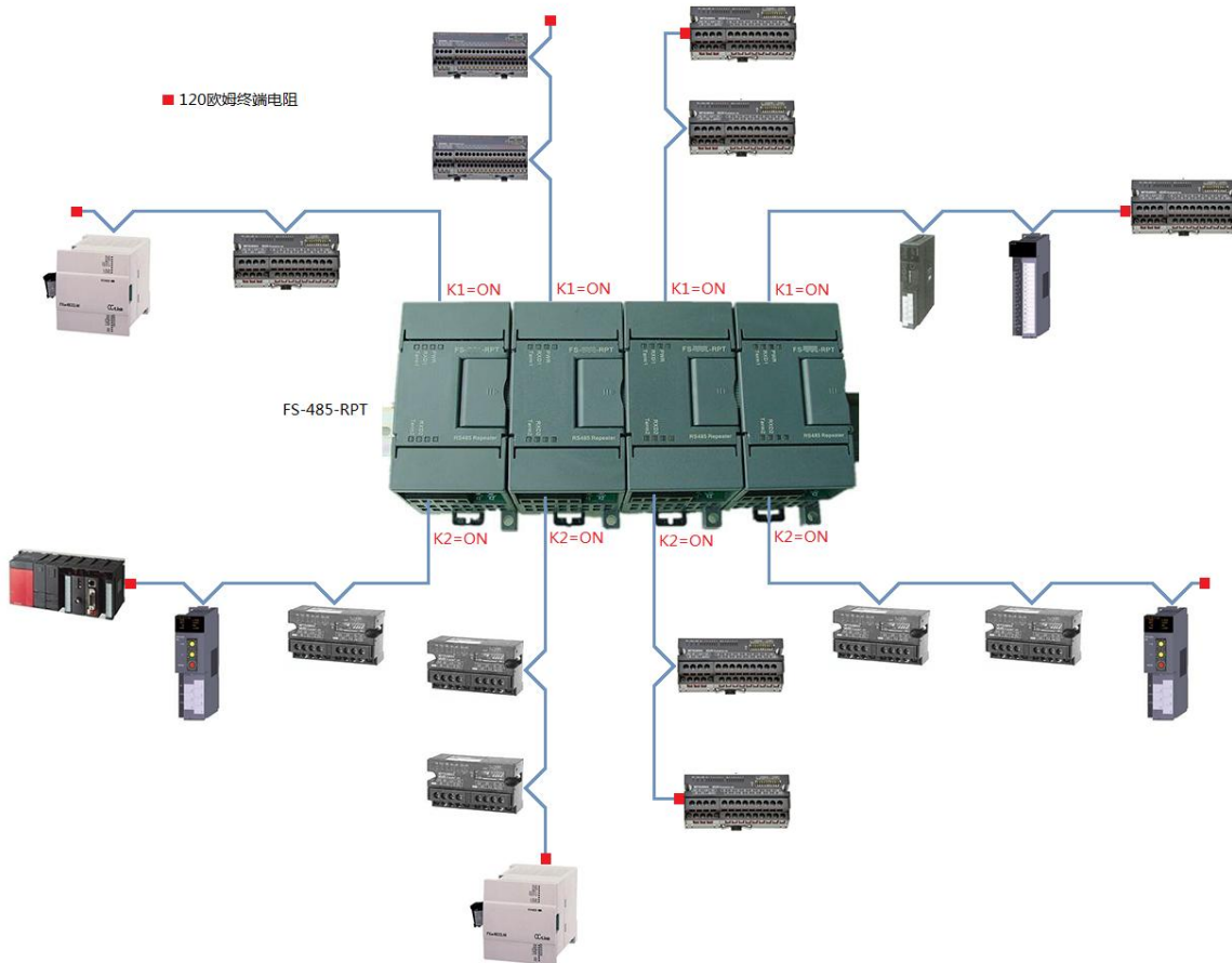
图 6-4 FS-485-RPT 组成集线器的网络拓扑
