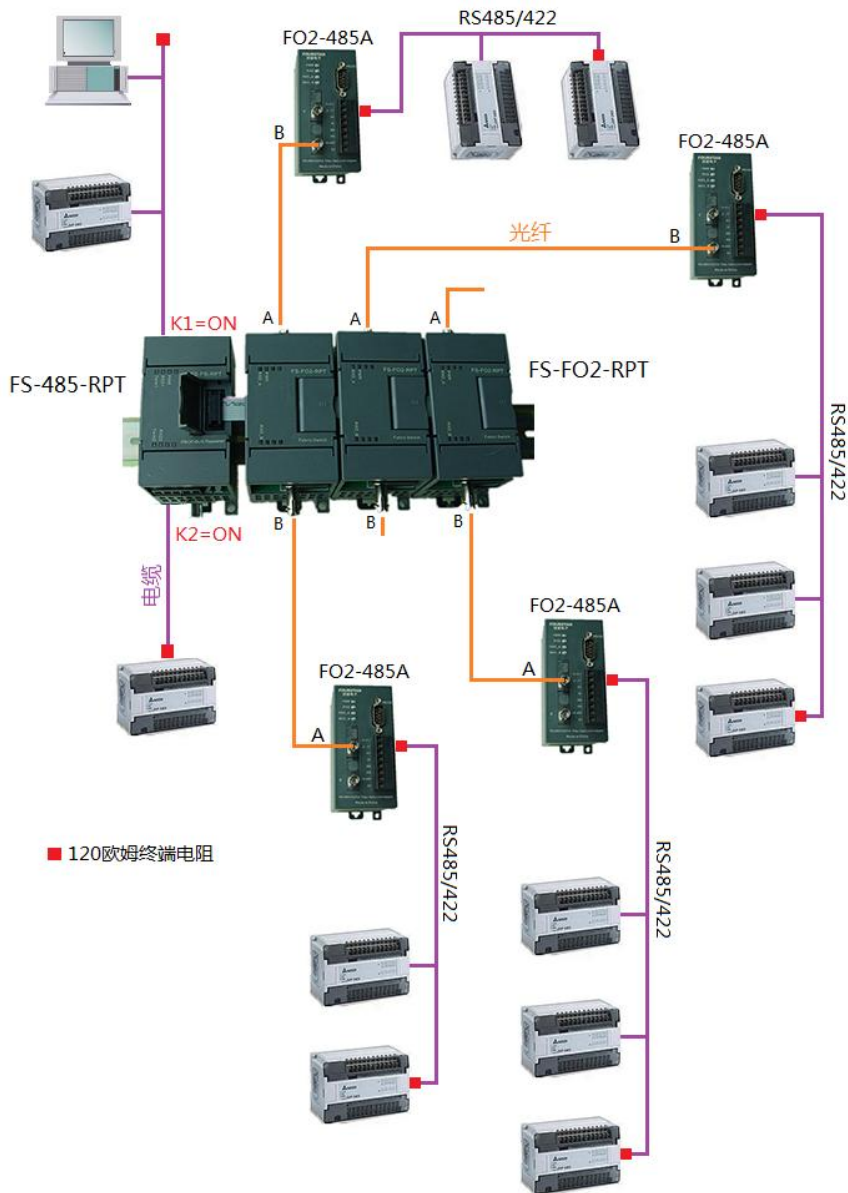
图 6-3 RS485 电缆和光纤混合网络
