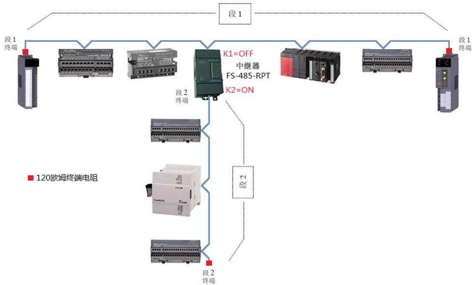
图 6-2 用 FS-485-RPT 中继器实现总线分支
